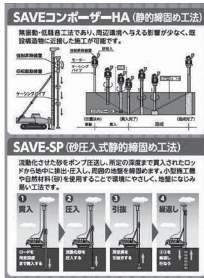
左：高潮堤防の地盤改良工法（葭ヶ須工区①②）
